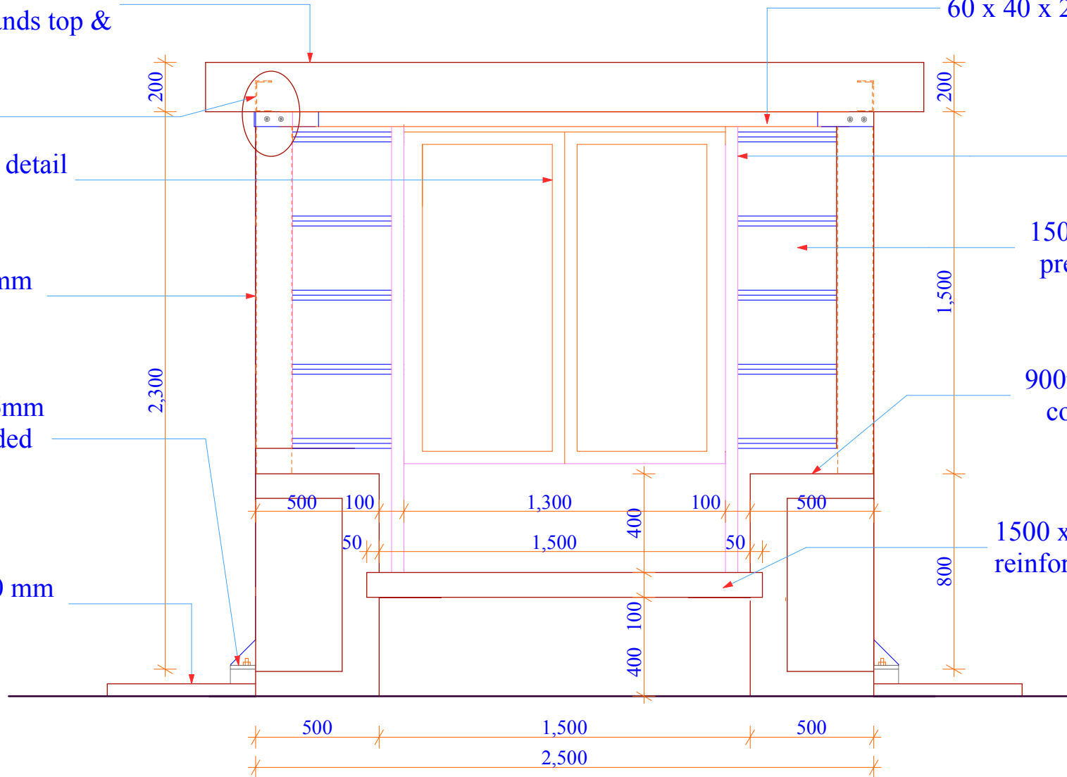
ELEVATION 02
